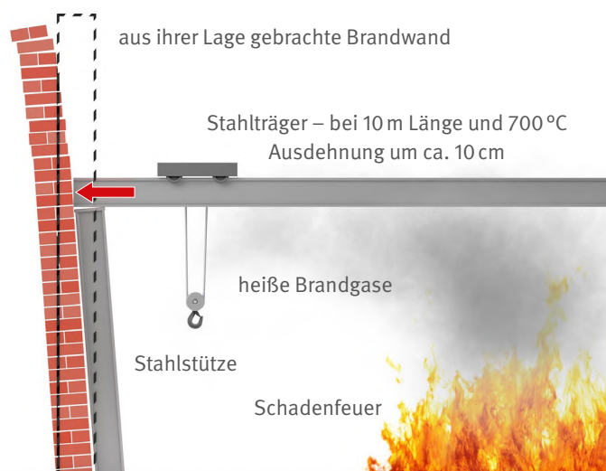
Abb. 8 Die Schubkraft eines erwärmten Stahlträgers kann eine Wand zum Einsturz bringen
